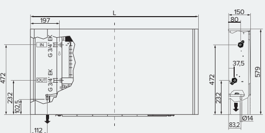
Instalare pe podea
